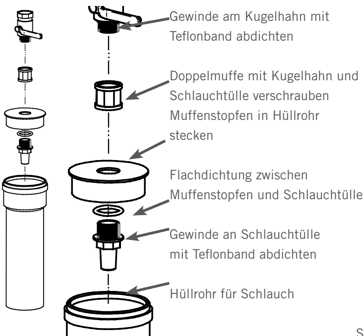
Montage Einzelteile
