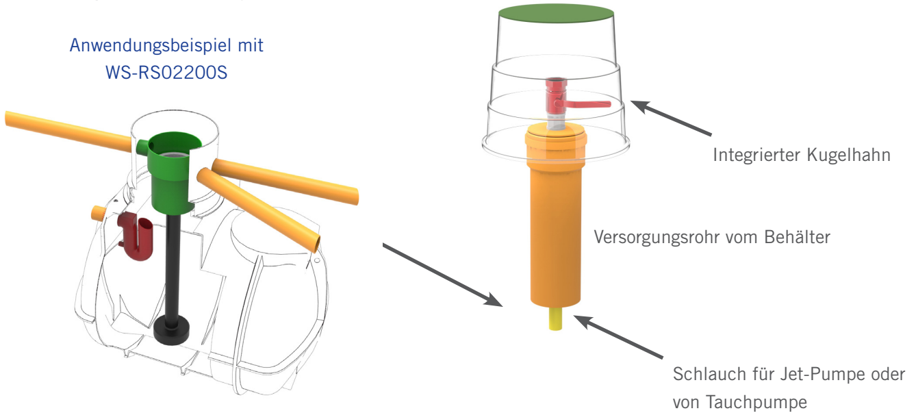
Montage Einzelteile
