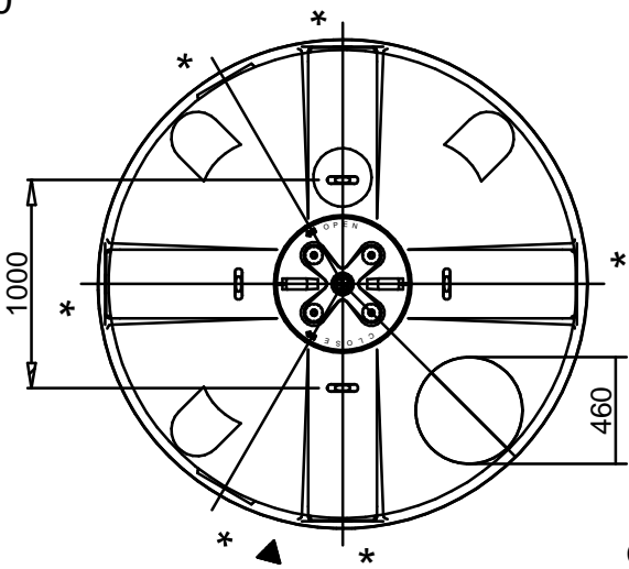
obere Flachstelle halbrund
